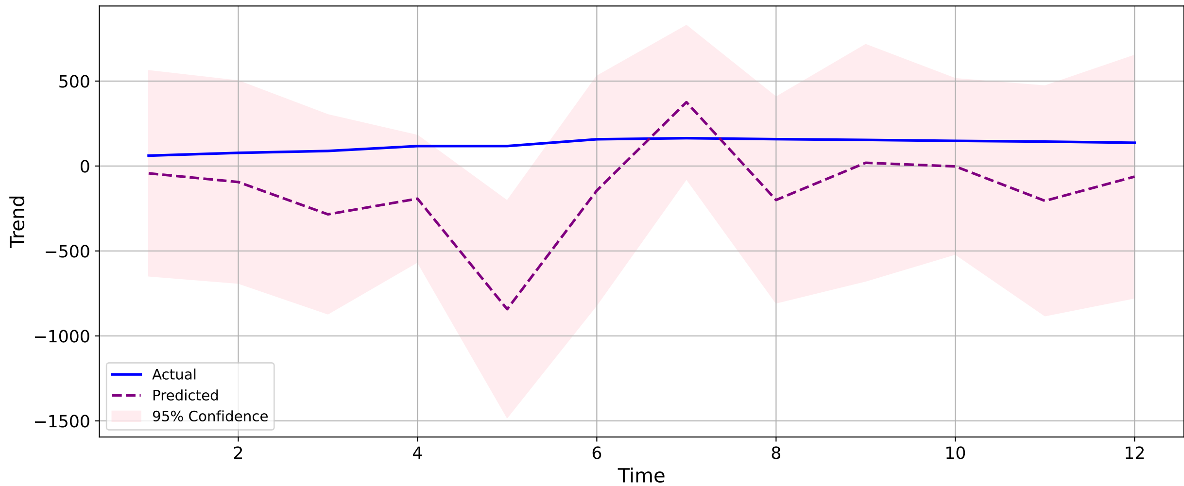
Trojan-ALL - Validation
